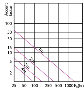
LEDspots 20W AR111 G53 927 40D
